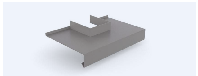
Pfostenausschnitt 3-seitig fertig geklebt bei Kleinteilen, max. 50 cm Schenkellänge
